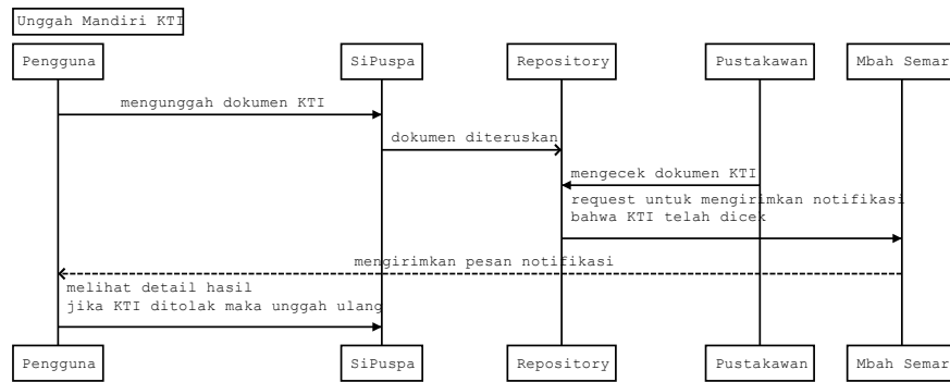
Gambar 2. 3 Diagram alur fitur unggah mandiri karya di dalam SiPuspa
